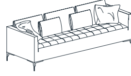
180 SM KOLTUK L: 1800 mm D: 870 mm H: 829 mm
